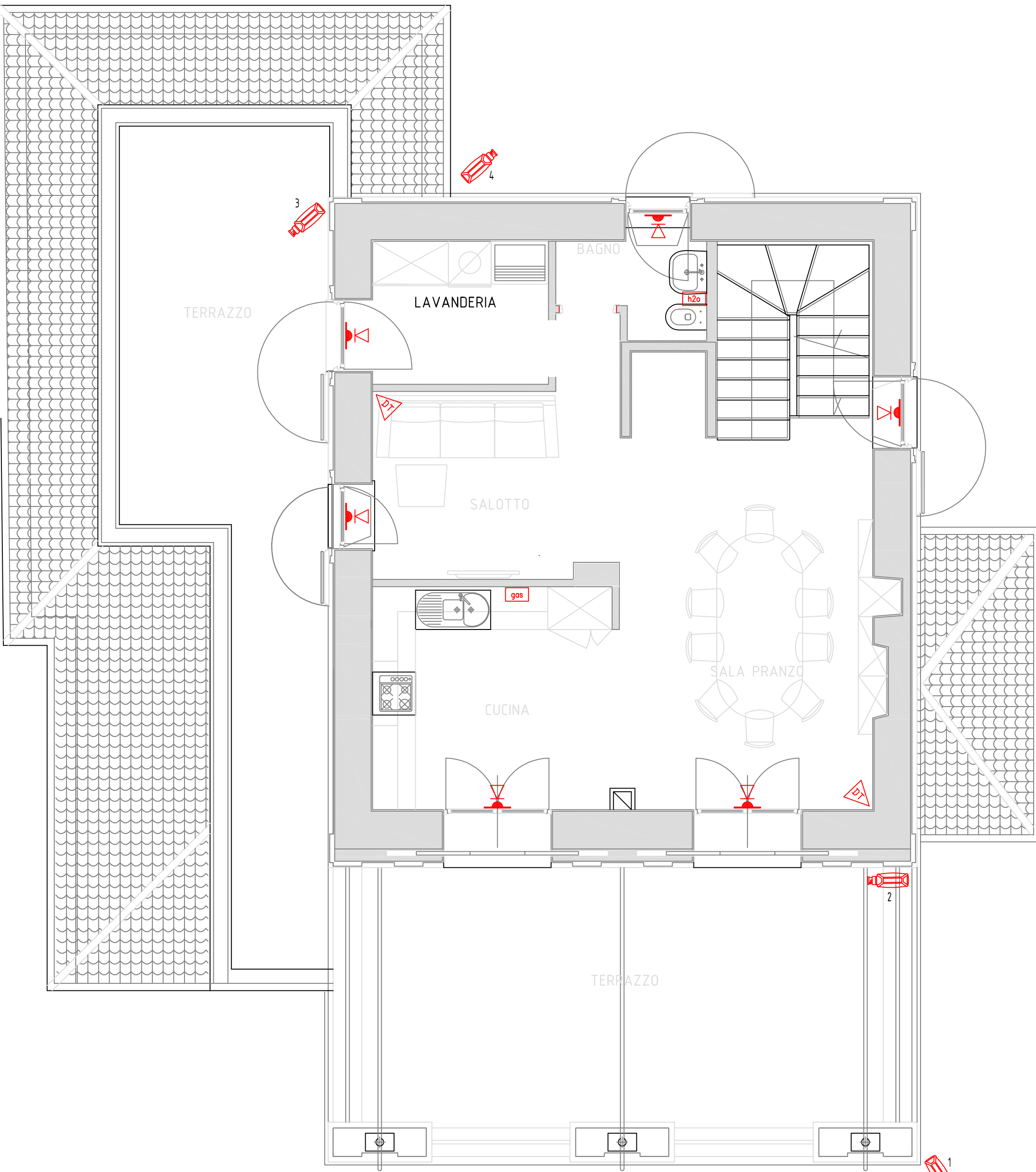
PIANTA PIANO PRIMO scala 1:50 IMPIANTO ANTITRUSIONE/TVCC REV. 5/3/2012
